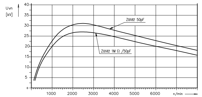
CHARAKTERISTIKA VYSOKÉHO NAPĚTÍ(HIGH VOLTAGE CHARACTERISTIC)
