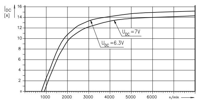
PROUDOVÁ CHARAKTERISTIKA SOUPRAVY(POWER CHARACTERISTIC)
